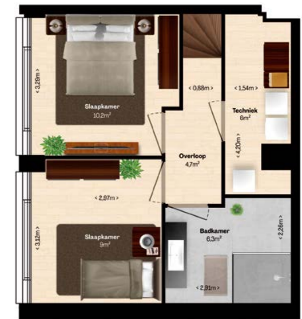
Appartement 3 Benedenverdieping
