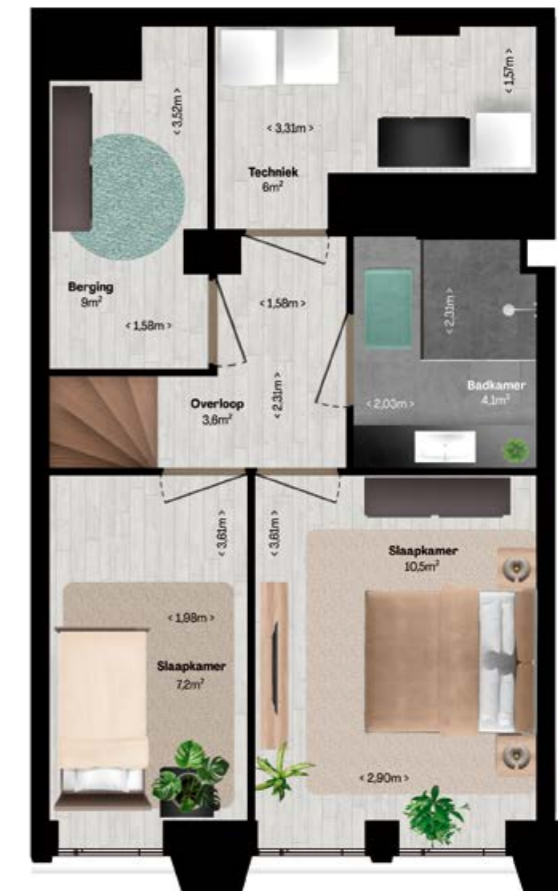
Appartement 11 Entresol
