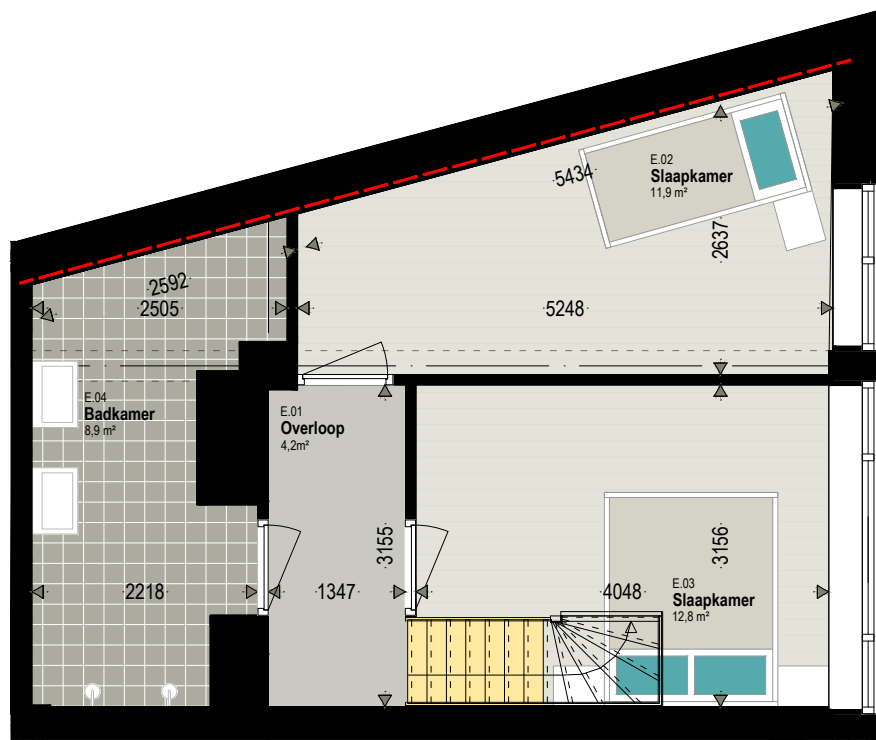
ENTRESOL
