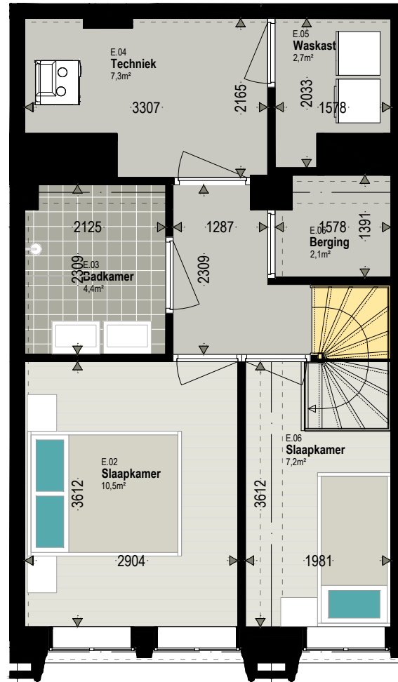
ENTRESOL
